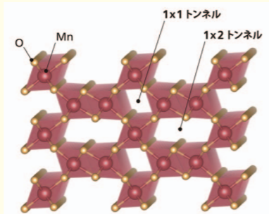
図2 γ-MnO 2 の結晶構造(断面図) 1x1トンネル構造と1x2トンネル構造、2種類の隙間構造を持つγ-MnO 2 。
