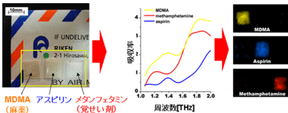
図2 郵便物中の薬剤の同定
