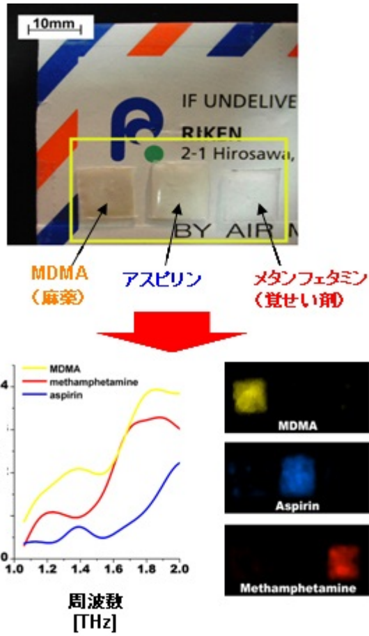
図 封筒に隠した薬剤をキャッチ
