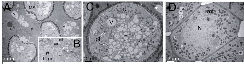
図4 電子顕微鏡 TEM で撮影したゼンソウのミトコンドリア
