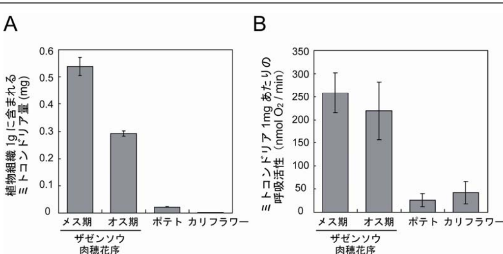
図5 発熱植物ゼンソウと非発熱植物（ポテト、カリフラワー）との比較。
