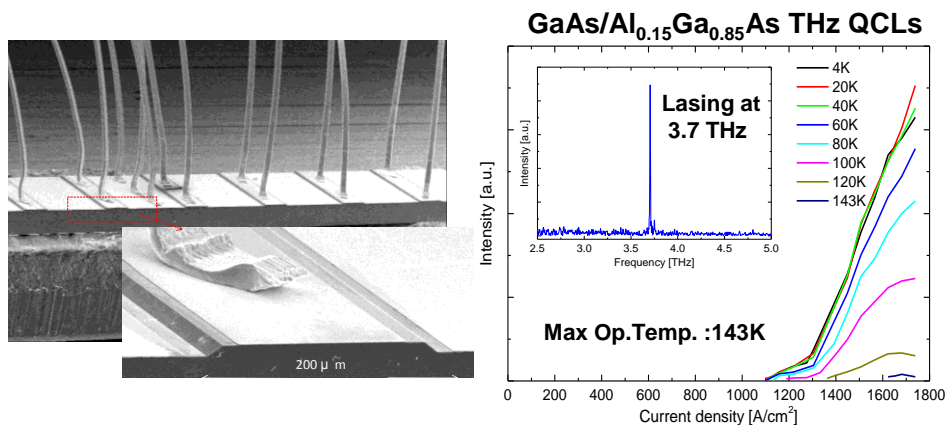
図4. GaAs 系テラヘルツ量子カスケードレーザーの素子概観と発振動作特性
